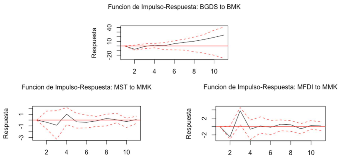
Figura 2: Análisis impulso respuesta.
