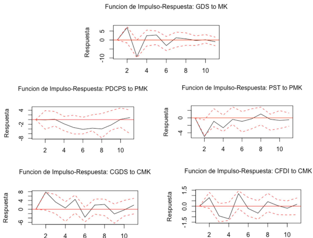
Figura 1: Análisis impulso respuesta.
